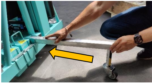
Zdjęcie 10. Wsuwanie obróconego stabilizatora
