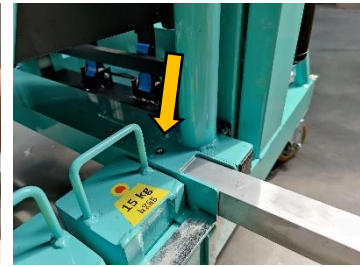
Zdjęcie 12. Zablokowany bolec zabezpieczający
