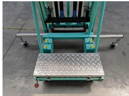
Zdjęcie 13. Rozłożone stabilizatory
